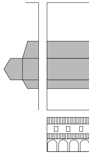
Ab-3 Tre cellule in larghezza su due livelli, con aggiunta sul retro e loggiato
