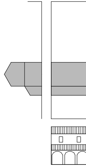
Aa-6 Bicellula in larghezza su due livelli, con loggiato
