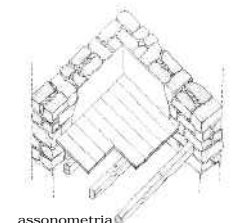
assonometria
