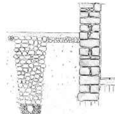
vespaio o drenaggio non aderente alla muratura
