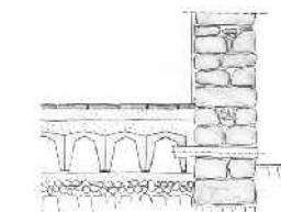
intercapedine orizzontale con elementi a igloo
