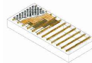
spaccato assonometrico
