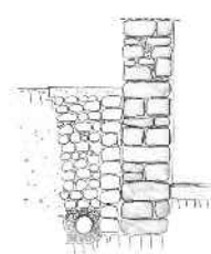
vespaio o drenaggio aderente alla muratura
